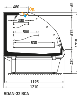
RDAN-32 BCA
